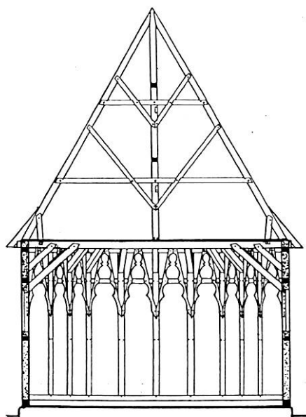
przekrój poprzeczny
