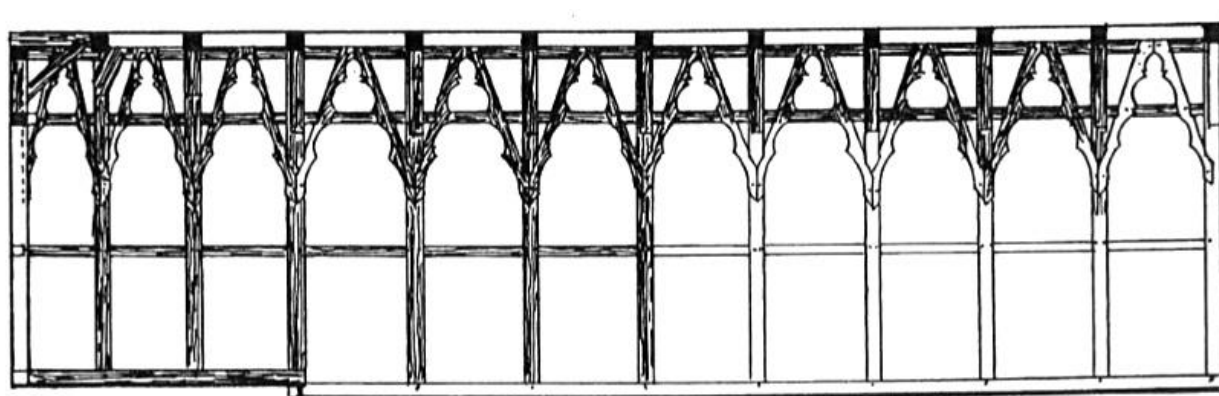
ściana południowa
