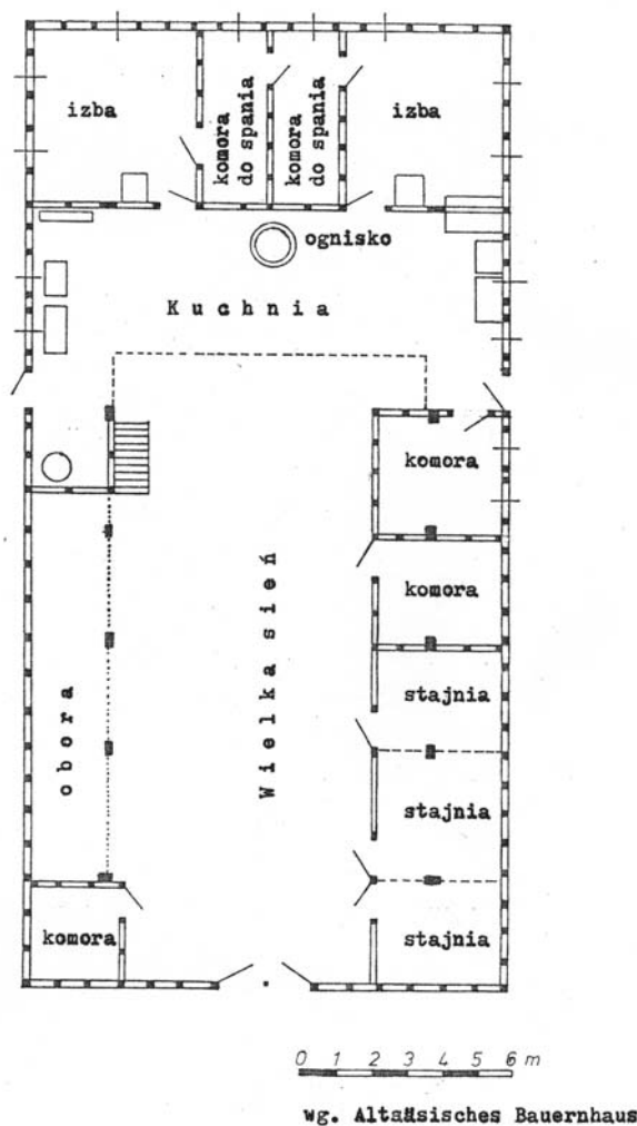
il. 1. Plan typowej chałupy saskiej
